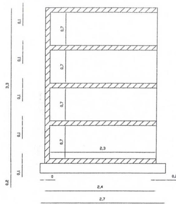
Sezione Longitudinale
