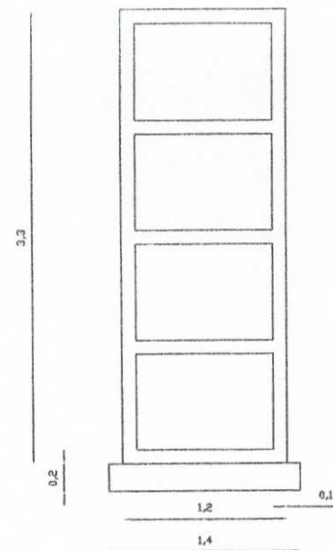
Prospetto Frontale
