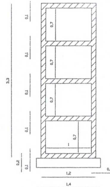
Sezione Trasversale
