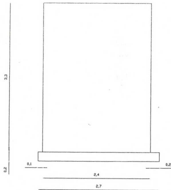
Prospetto Laterale
