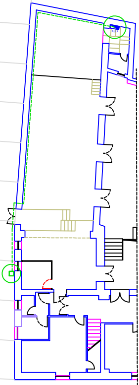
PLANIMETRIA IMPIANTO MESSA A TERRA 1:100
