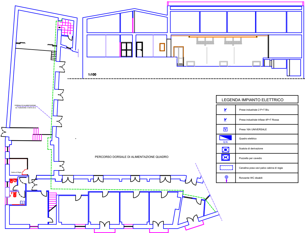
PLANIMETRIA IMPIANTO ELETTRICO 1:100
