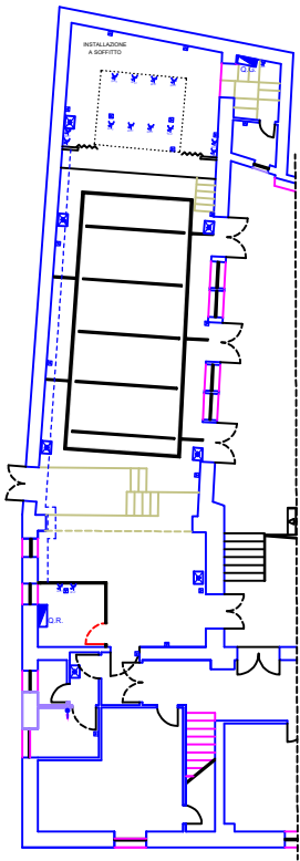
PLANIMETRIA IMPIANTO ELETTRICO 1:100
